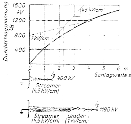
Abb. 14. Endstadien der Vorentladung bei s = 1 m und 4 m
