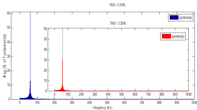
Fig. 19 Courant THD
