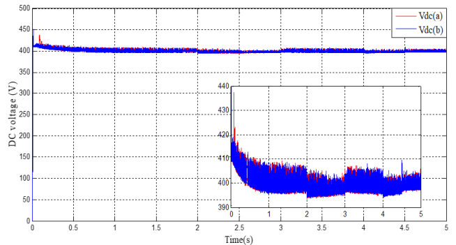
Fig. 17 DC voltage
