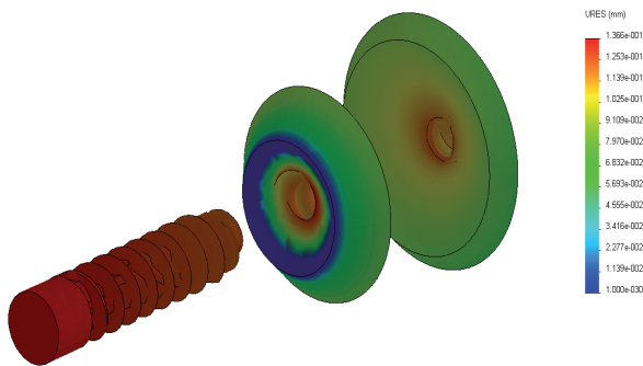
Fig. 9 Displacement of linked elements (URES: Resultant Displacement – equipollent displacement)
